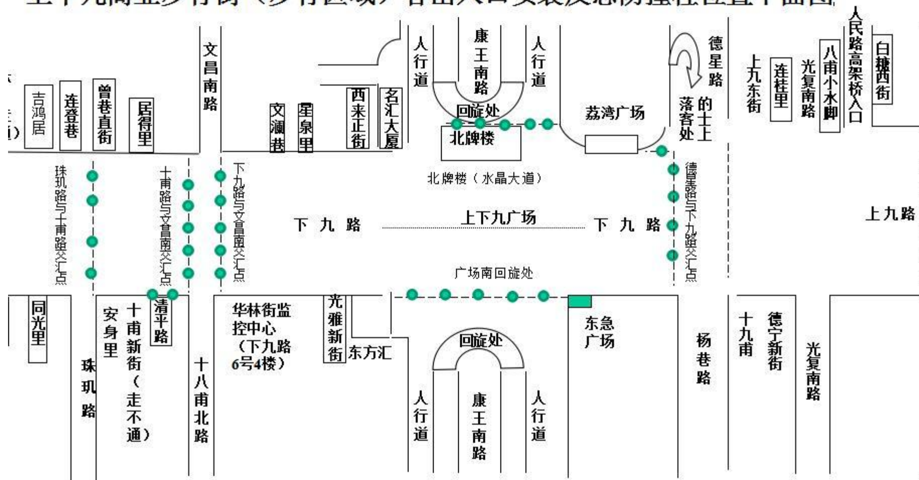
上下九商业步行街（步行区域）各出入口安装反恐防撞柱位置平面图
